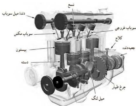
طرحی از اجزای درونی یک ماشین بنزینی
