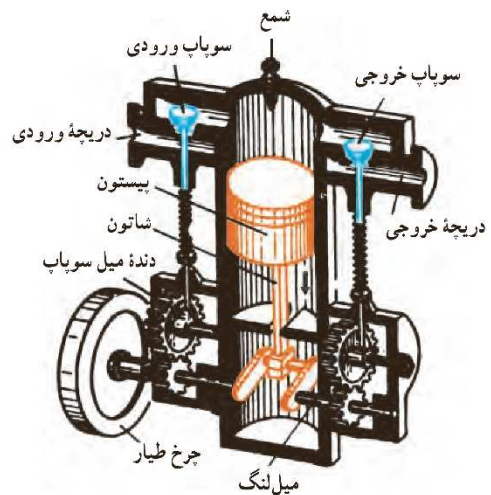
استوانه (سیلندر) و اجزای جانبی موتور
