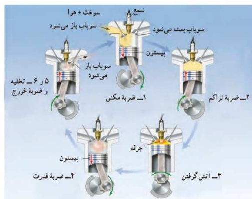
مراحل مختلف در چرخه موتورهای درون‌سوز
