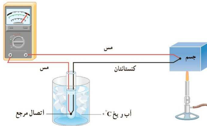
طرحی از یک دماسنج ترموکوبل
